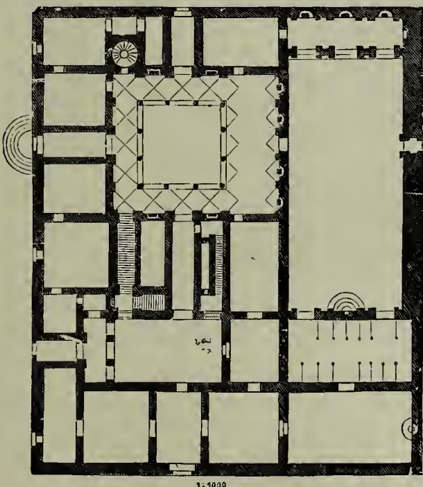
Abb. 192. Pal. Riccardi zu Florenz. Grundriß.
